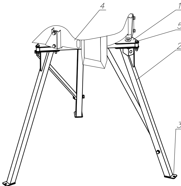
Рис. 10 Опора смесителя.
