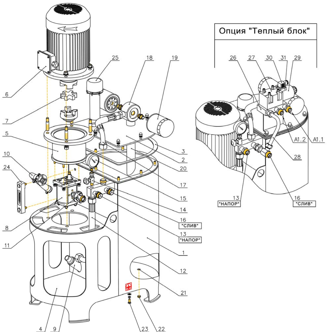
Рис. 5. Установка насосная.
