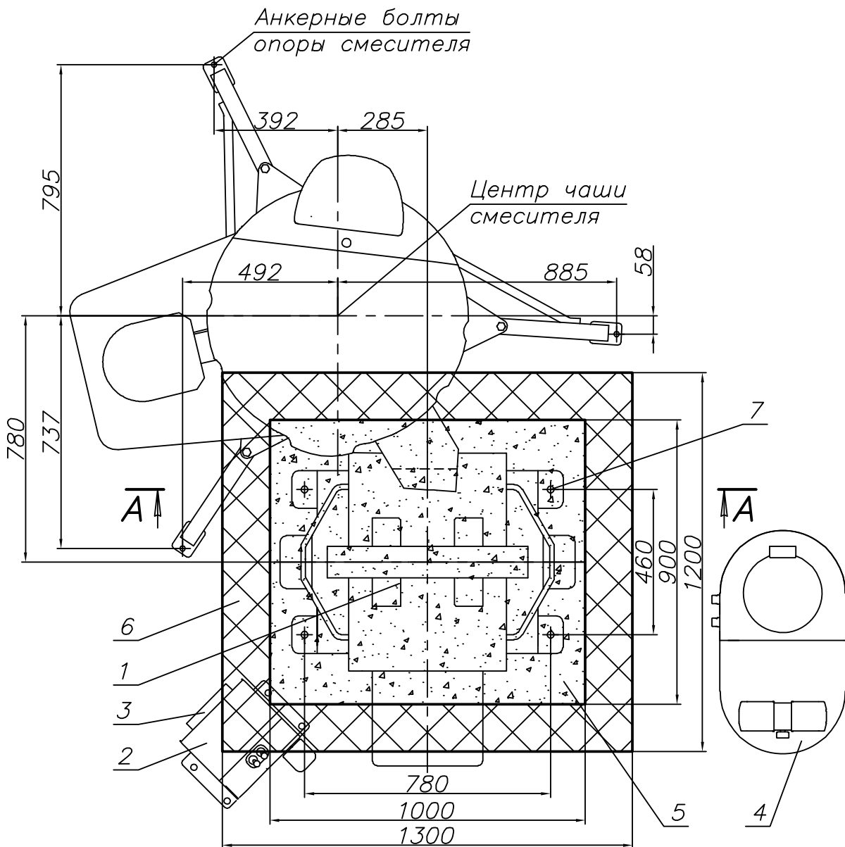
Рис. 13. План фундамента.
