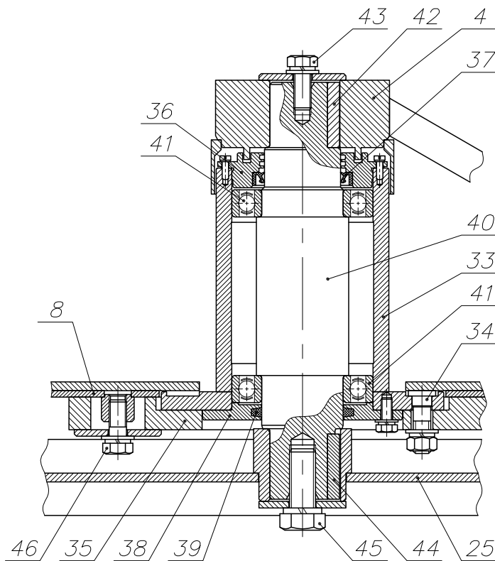
Рис. 9. Опора ротора.
