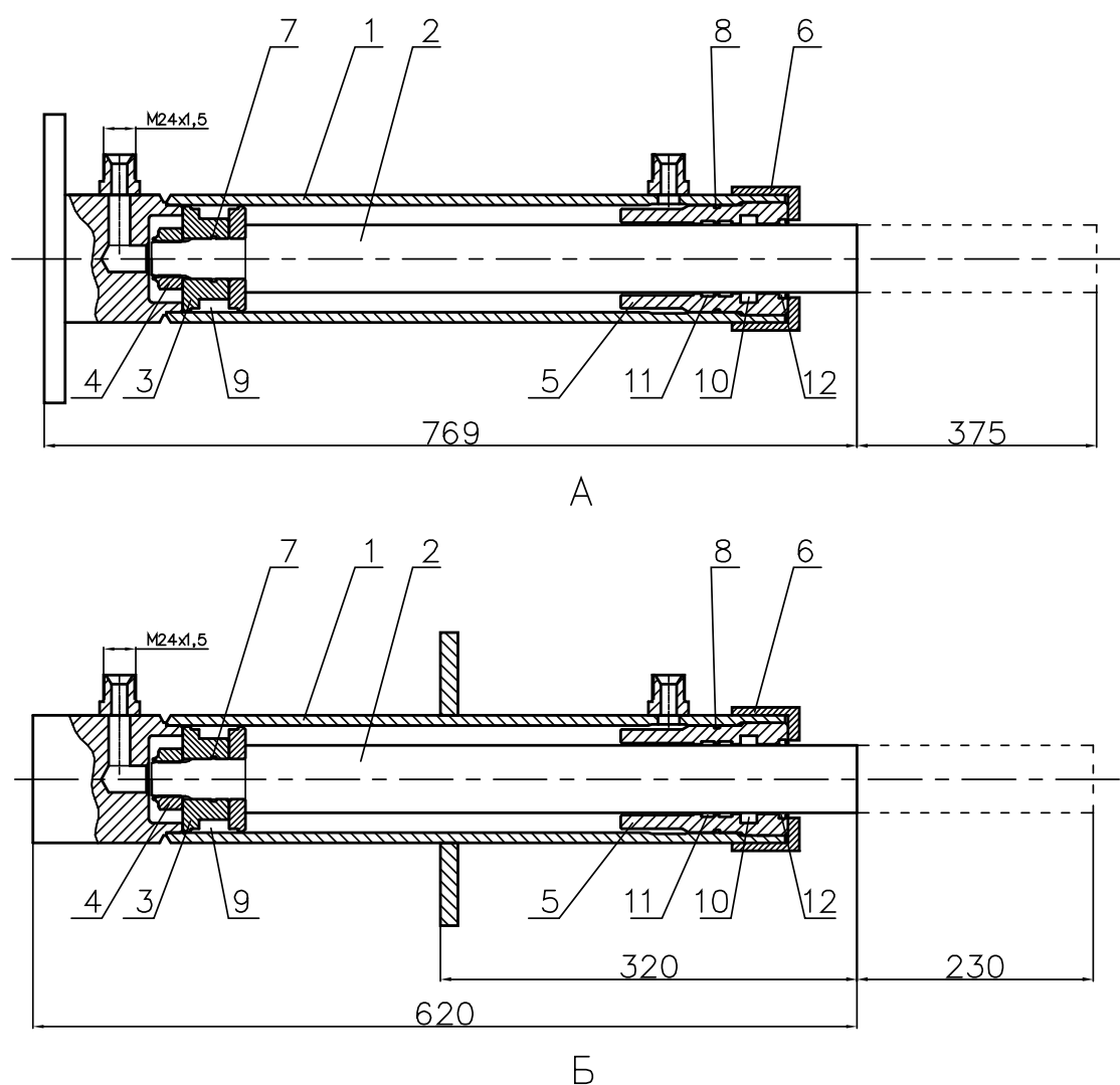
Рис. 7. Гидроцилиндры.
