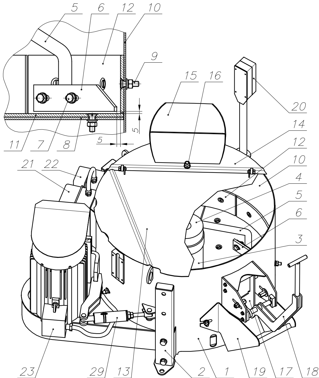
Рис. 8. Смеситель, вид сверху.
