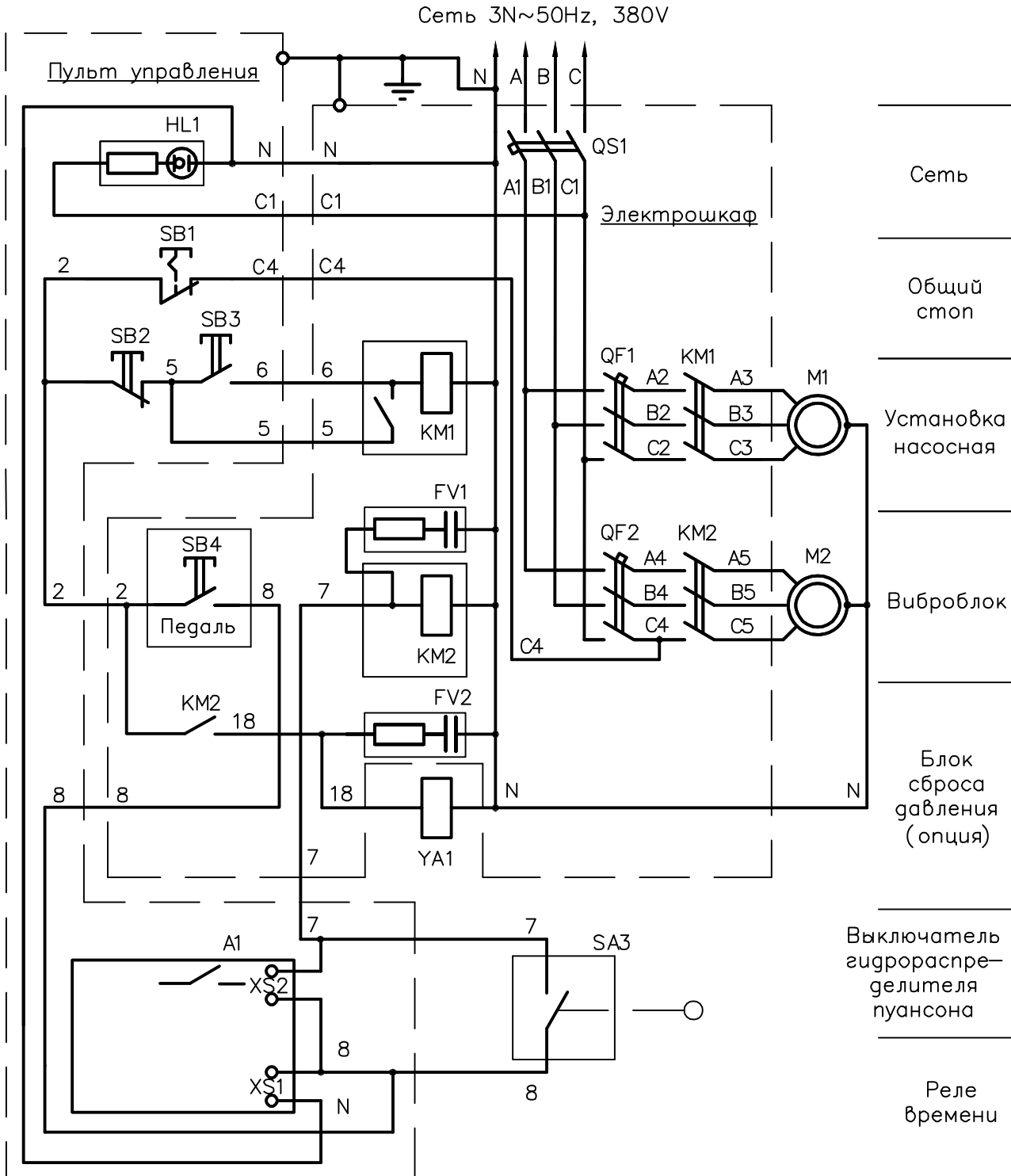
Рис. 11 .Схема электрическая принципиальная.
